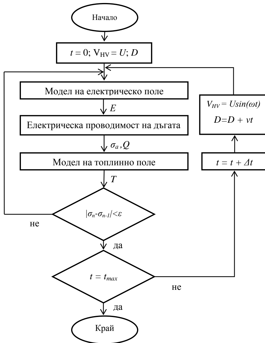
Фиг.2 Блокова схема
