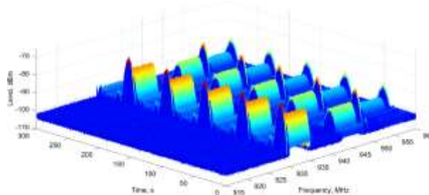
Фиг. 3. Периодично повтарящ се спектър при многооборотна ротация на сканиращата антена
