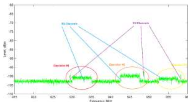
Фиг. 2. Спектрална картина в диапазона 915 ÷ 960 MHz
