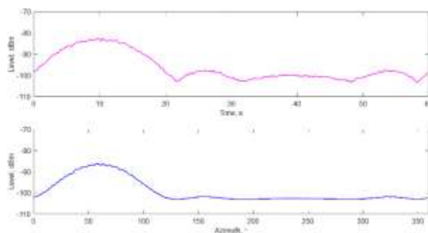
Фиг. 6. Периодично повтарящо се ниво за честота 932,5 MHz в интервала 0 \div 60s ( 0^\circ \div 360^\circ )
