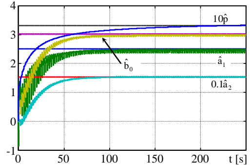
Figure 6: Parameter estimation
