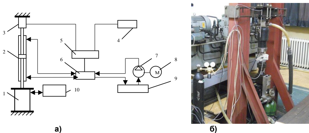
Фиг. 2. Схема на стенда (а) и общ вид (б): 1 – еластичен елемент; 2 – хидравличен цилиндър; 3 – възприематели за сила и преместване; 4 – генератор на сигнал; 5 – управляващ блок; 6 – сервоклапан; 7 – помпа; 8 – ел. двигател; 9 – резервоар за масло; 10 – въздушен резервоар.
