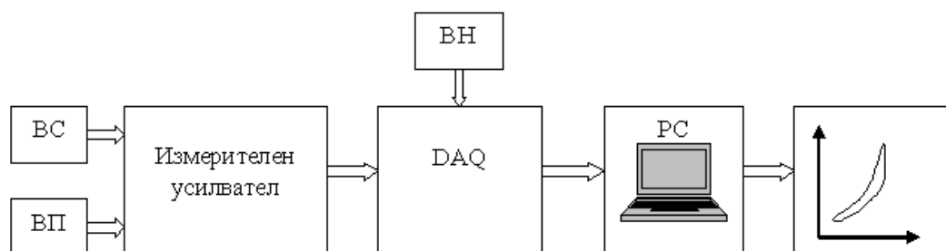
Фиг. 3. Блок-схема на измерителната верига: BC – възприемател за сила от тензорезисторен тип; BP – възприемател за преместване от индуктивен тип; BH – възприемател за налягане от тензорезисторен тип; измерителен усилвател – универсален тензометричен усилвател HBM – Scout 55; DAQ (Data Acquisition) – устройство за събиране на данни тип EspressoDAQ DQ 401 – HBM; PC – персонален компютър с инсталиран програмен продукт Catman – HBM.
